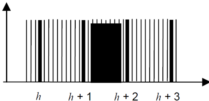
شکل ۲- نمایش گرافیکی مفهوم زیرگروه مرکزی هارمونیک میانی در طیف فرکانسی یک تابع زمانی
