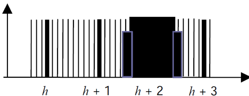
شکل ۱- نمایش گرافیکی مفهوم گروه هارمونیکی در طیف فرکانسی یک تابع زمانی
